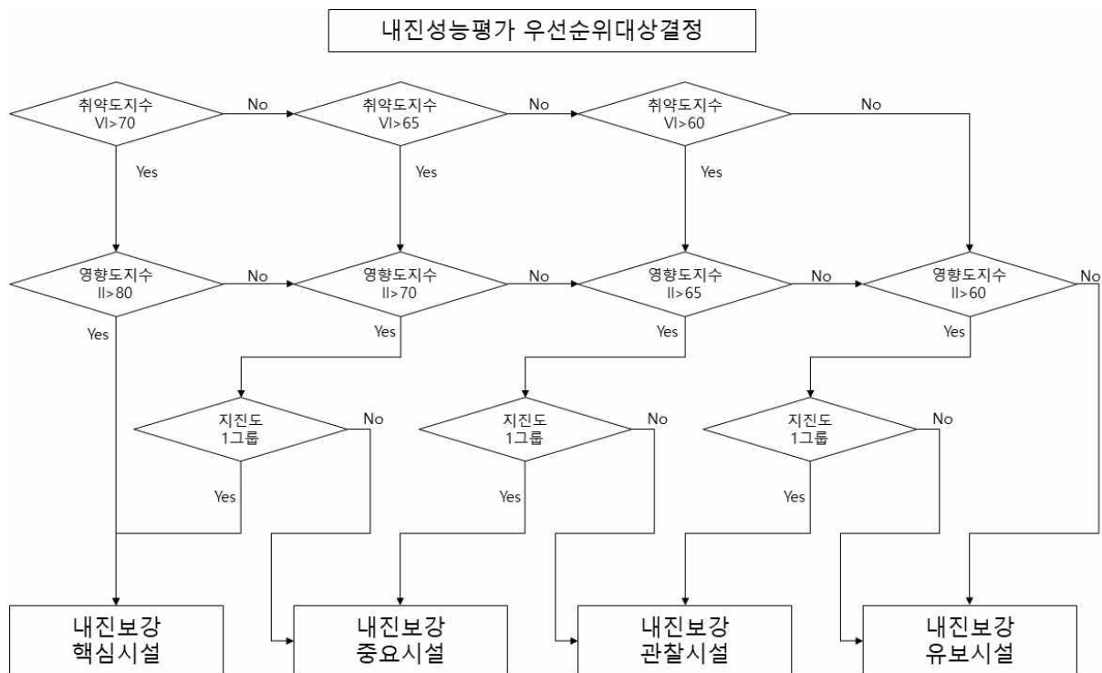
해설 그림 3.4.2 내진그룹화 방법
