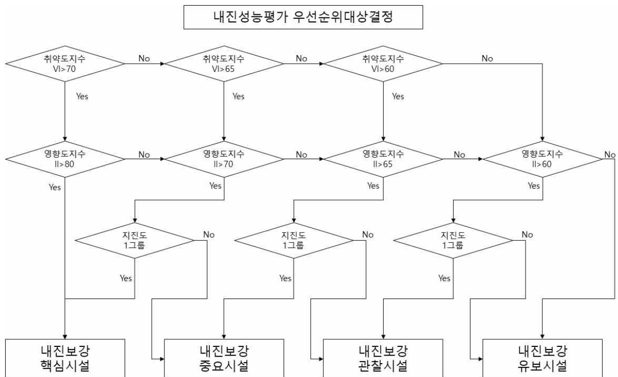
그림 B1.1 내진그룹화 방법
