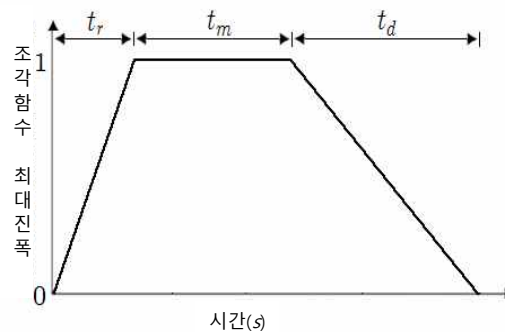
<그림 A.4> 가속도시간이력의 구간선형 포락함수
