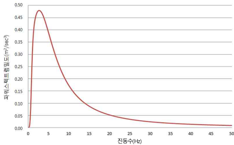
<그림 A.5> 수정 Kanai-Tajimi 모델의 형상
