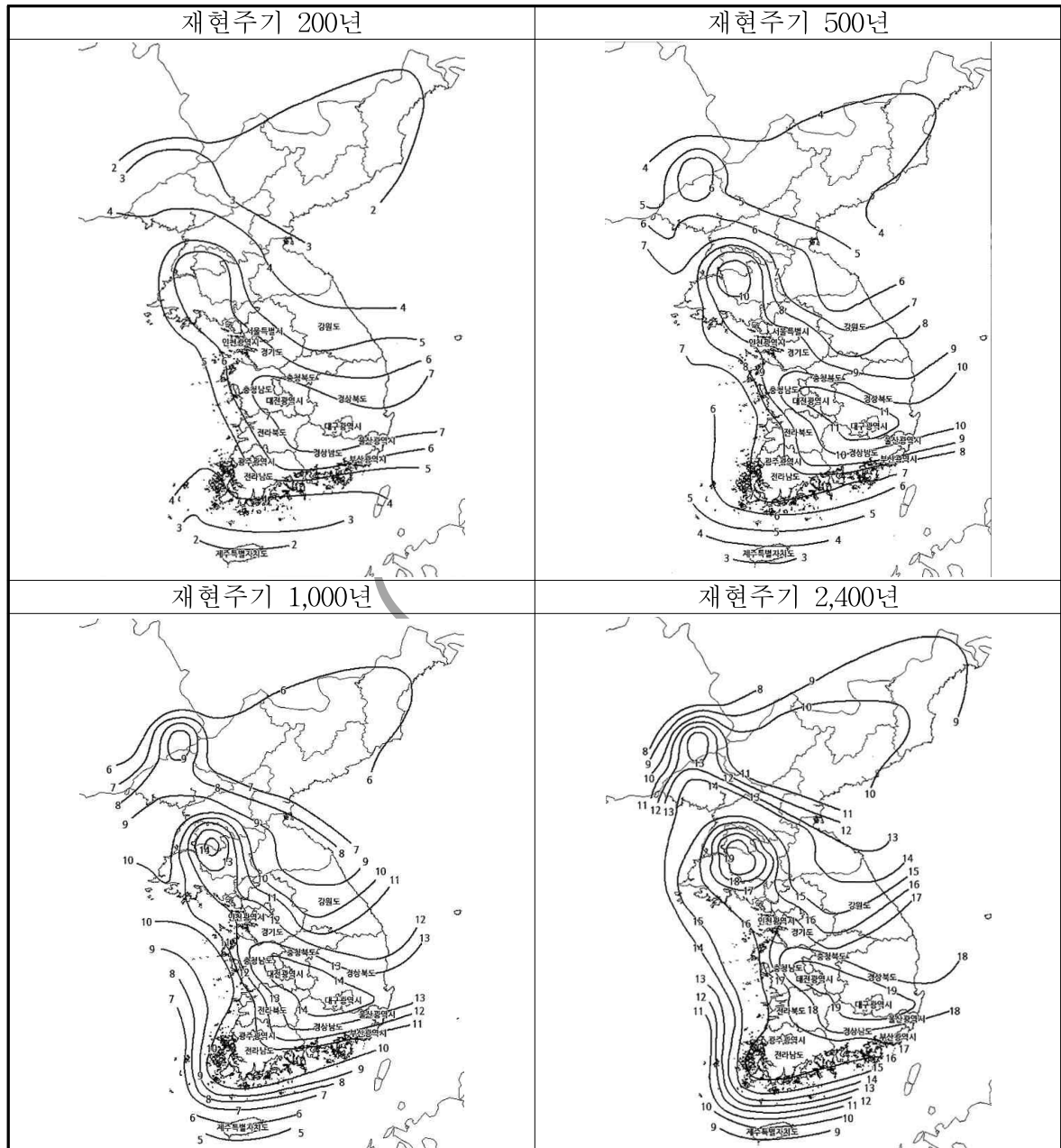
해설 그림 2.2.1 국가지진위험지도(소방방재청, 2013)
