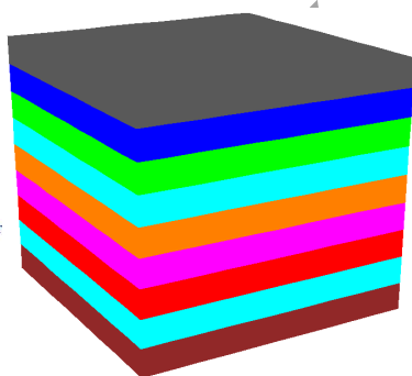
a) 초기 전단탄성계수 분포도
