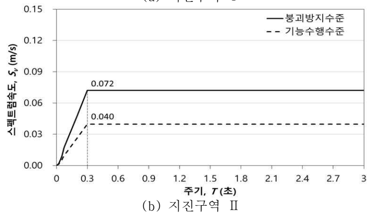
해설 그림 2.2.3 기반면에서의 설계속도응답스펙트럼
