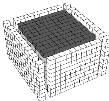
(b) Free-field 경계요소 반영
