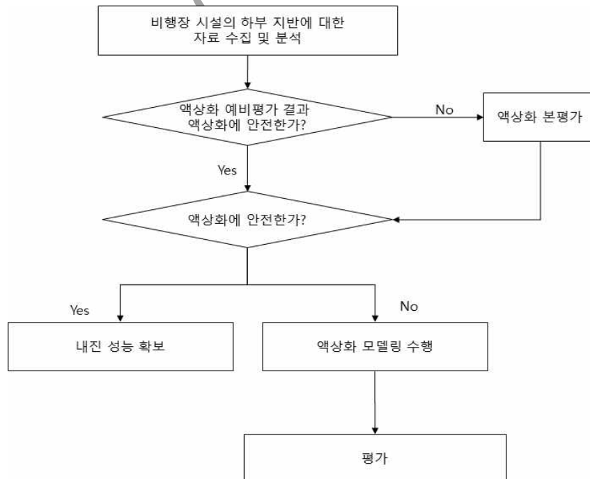
해설 그림 4.1.1 비행장 시설 내진성능 상세평가
