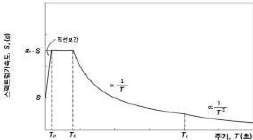
<그림 A.1> 암반지반 수평설계지반운동의 가속도 표준설계응답스펙트럼
