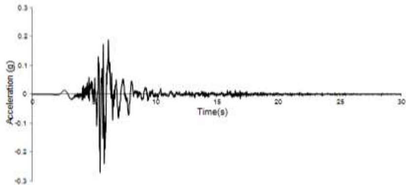
그림 B2.5 입력 지진 가속도-시간이력(붕괴방지수준, 2400년 재현주기)
