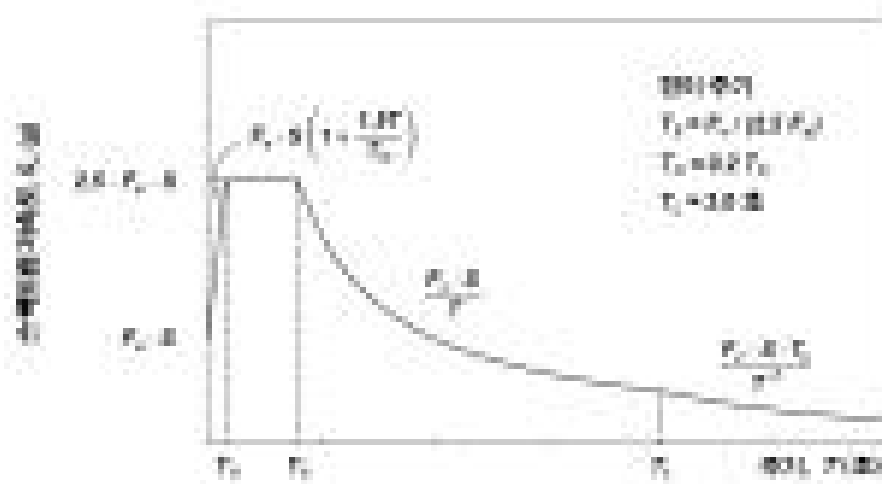
<그림 A.2> 토사지반 수평설계지반운동의 가속도 표준설계응답스펙트럼
