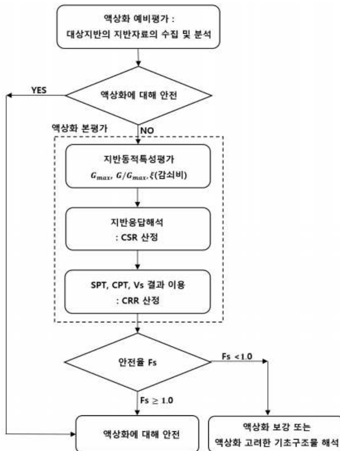
해설 그림 4.2.1 액상화 평가 흐름도
