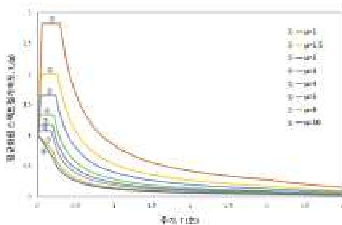
<그림 A.3> 표준설계응답스펙트럼에 대응하는 비탄성응답스펙트럼 기준 ( T=0.01 초에서 S_a=1g 로 정규화)
