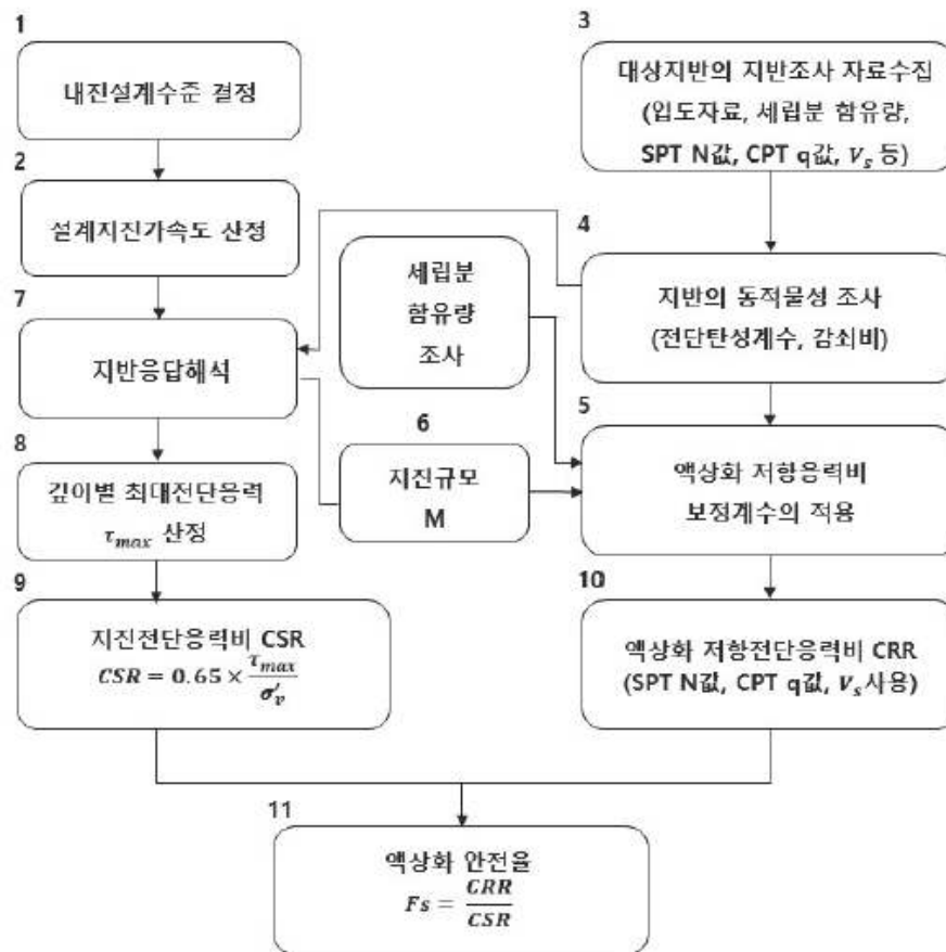
해설 그림 4.2.3 액상화 본평가 흐름도
