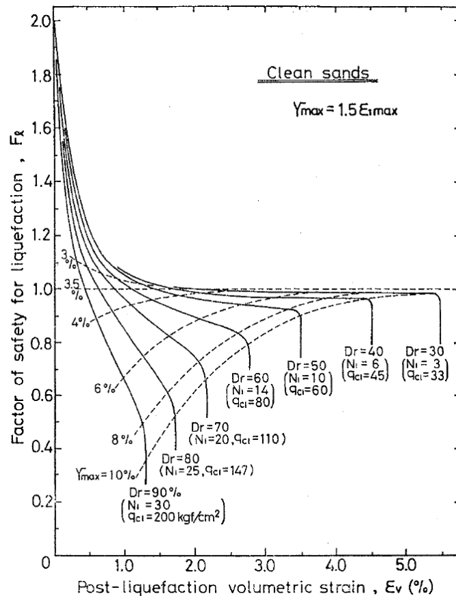
그림 B2.2 액상화 안전율에 따른 부피변형률 결정(Ishihara & Yoshimine, 1992)
